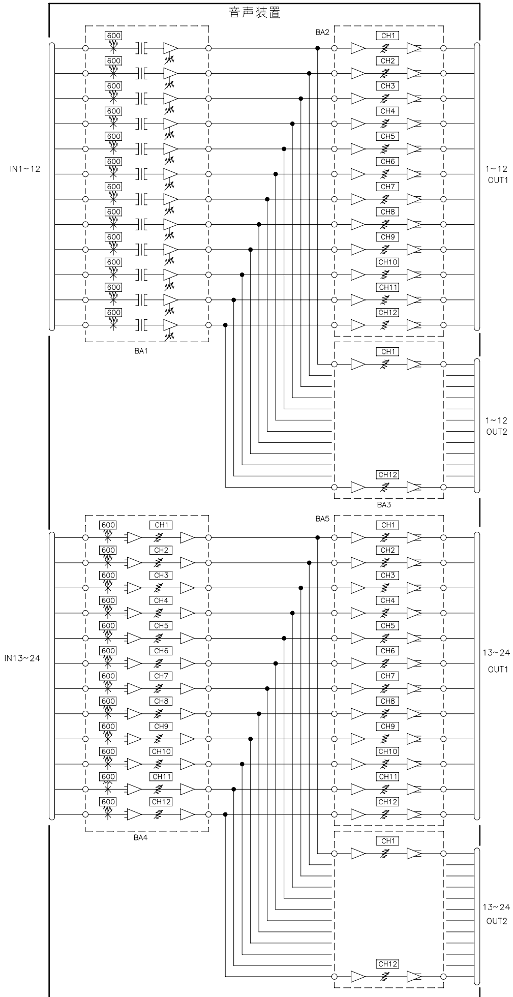
(参考) 音声系統図
